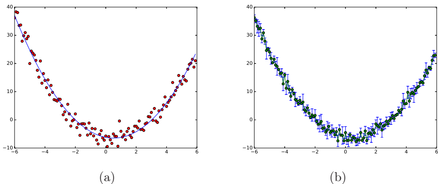
Рис. 7. Иллюстрации к задачам 24 — (a) и 25 — (b). На рис. (a) представлена зависимость y_i = x_i^2 - x_i - 6 + \xi_i (серые точки), где \xi_i — нормально распределённые случайные числа (шум) с нулевым средним и среднеквадратичным отклонением 2, и её аппроксимирующая функция (чёрная кривая), рассчитанная методом наименьших квадратов. На рис. (b) — зависимость \langle y_k(x) \rangle_{k=1,2,3} с разбросом ошибок, построенная по 3 экспериментам ( k — номер эксперимента), исходная зависимость сгенерирована по формуле y_i = x_i^2 - x_i - 6 + \xi_i , причём для каждого эксперимента реализация шума \xi своя.
