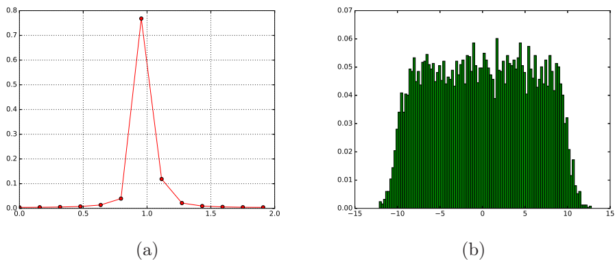
Рис. 8. Спектр мощности синусоиды, построенный по 1 периоду при шаге выборки \pi/12 — (a) и гистограмма сложного (суммы равномерного и нормального) распределения — (b).
