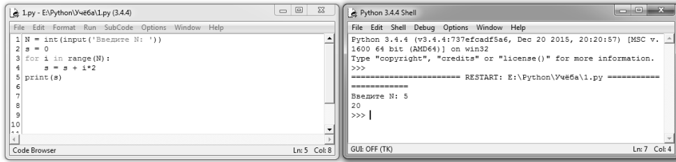
Рис. 3.3. Пример логической ошибки, которая может быть выявлена только разработчиком.
