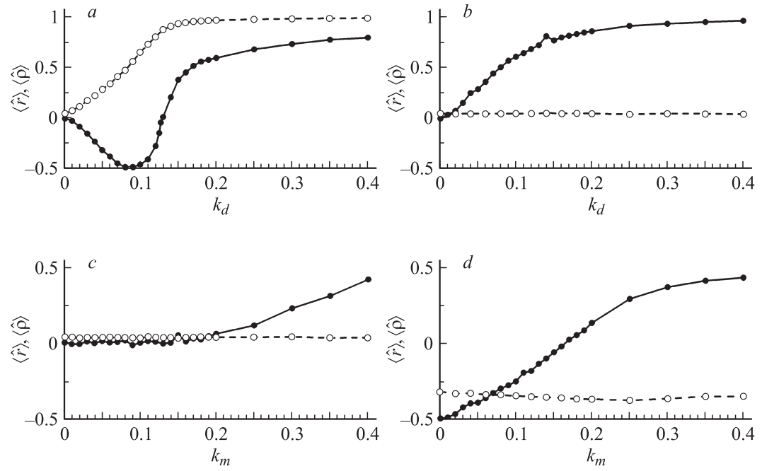
Рис. 2. Зависимость коэффициентов фазовой когерентности (штриховые линии) и корреляции приращения фаз (сплошные линии) от коэффициентов связи для a — синхронизирующей связи, b — разностной антисимметричной связи, c, d — модулирующей связи при b = 0 ( c ) и b = 0.7 ( d ).
