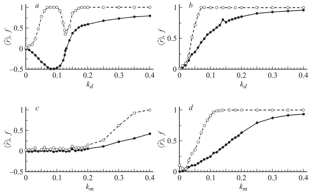
Рис. 1. Средние значения \langle \hat{r} \rangle (сплошные линии) и частоты положительных выводов f (штриховые линии), рассчитанные по ансамблю из 100 временных рядов: a — разностная связь с k_{d,1} = k_{d,2} = k_d , b — разностная связь с k_{d,1} = -k_{d,2} = k_d , c — модулирующая связь при b = 0 , d — модулирующая связь при b = 0.7 .
